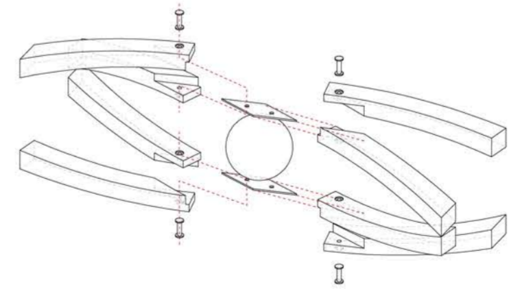
Esploso nodo centrale Exploded axonometric view central node SCALA 1:10
