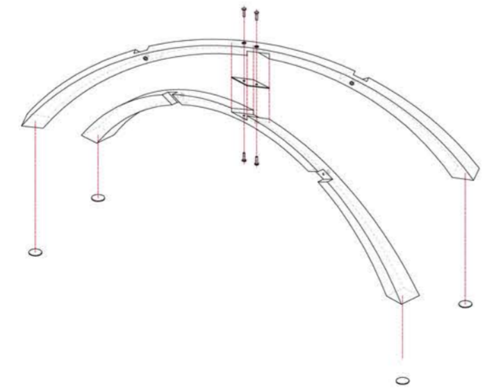
Esploso assometrico montaggio piastra Exploded axonometric view plate mounting SCALA 1:20
