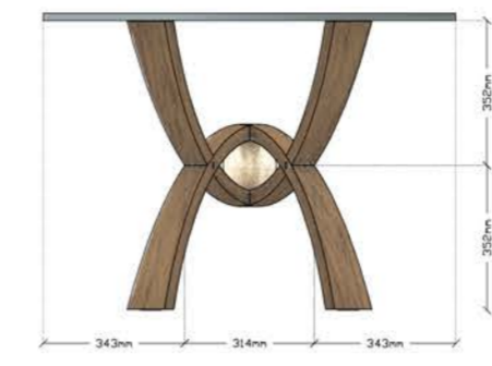
Prospetto laterale - Side elevation SCALA 1:20
