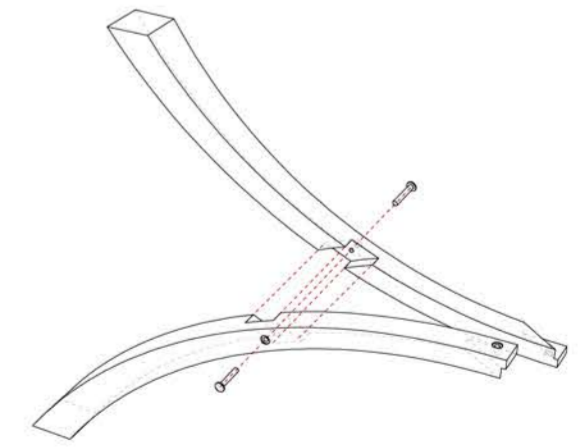
Esploso nodo esterno Exploded axonometric view external node SCALA 1:10
