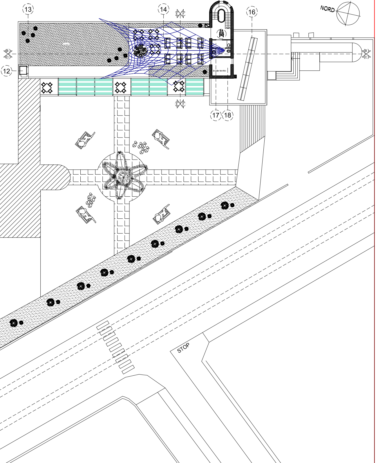
PLANIMETRIA GENERALE PIANTE TERZO LIVELLO-copertura Distribuzione interna ed arredo GENERAL PLAN THIRD LEVEL PLAN-coverage Internal distribution and furniture
